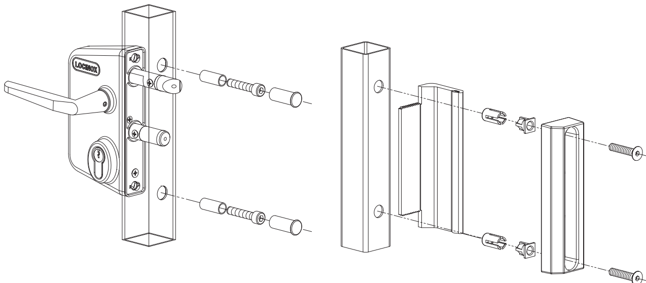
рис. 4 (для Сварных ворот и калиток)
